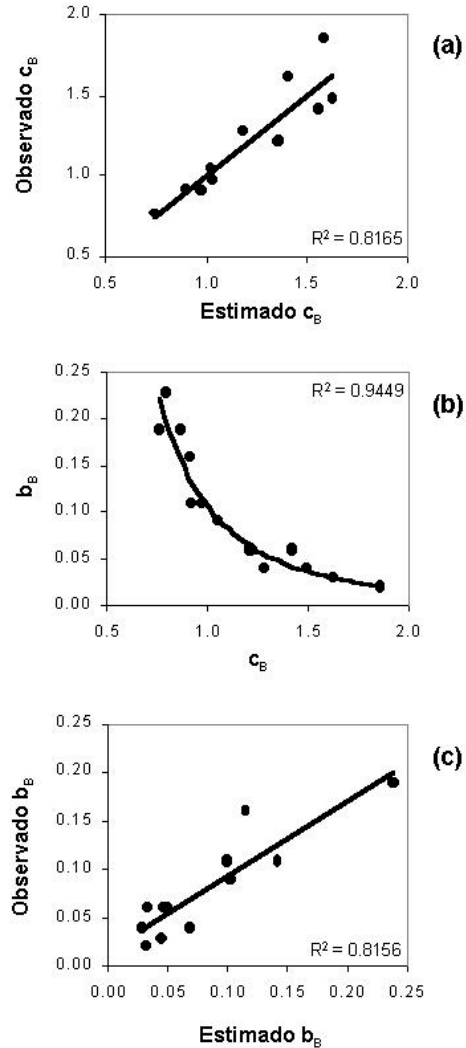
Figura 7: Relaciones entre valores observados y estimados para los coeficientes b_B y c_B del modelo Bristow-Campbell, y la relación entre ambos. (Baigorria et al. , 2003a)
