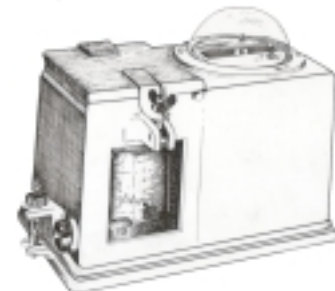
Figura 4. Actinógrafo o piranómetro bimetalico de Robitzch
